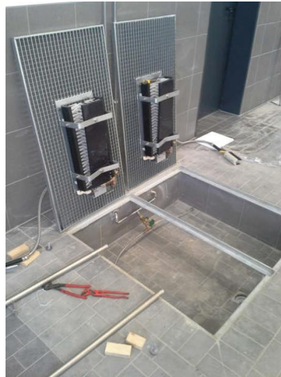
Rostenmaß der Stiefelwaschanlage: 830 mm x 520 mm
