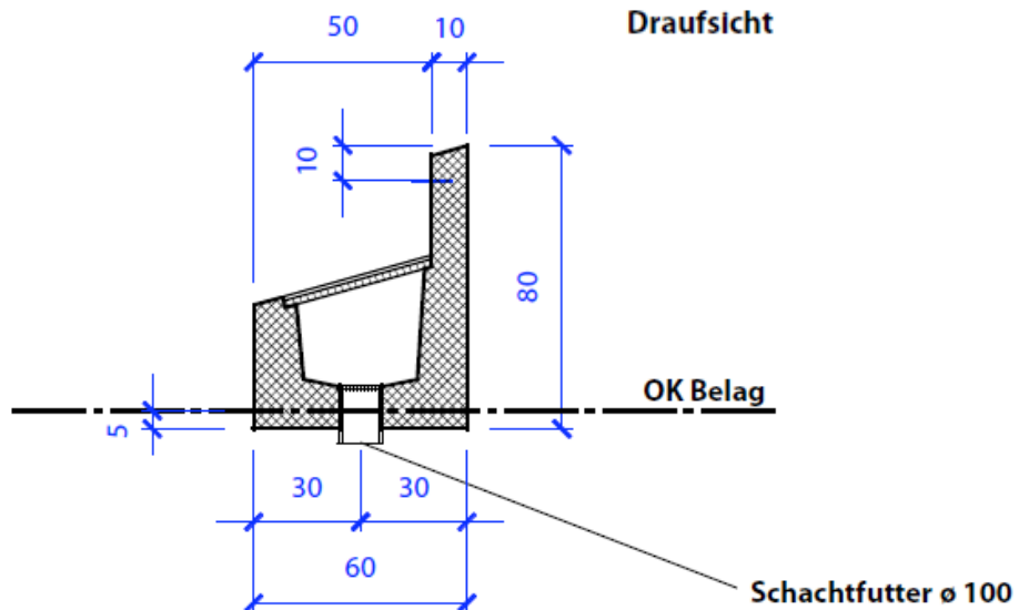
Querschnitt A - A
