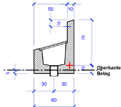
Coupe transversale de droite
