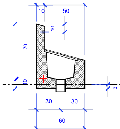
Coupe transversale de gauche
