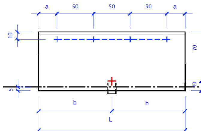
Vue du panneau arrière
